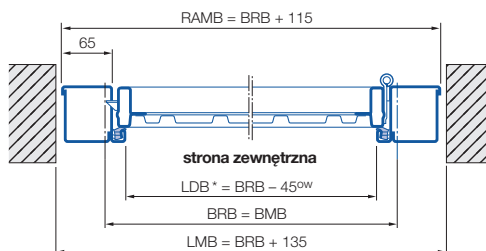
Montaż w otworze / otwieranie do wewnątrz
