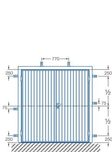
Rozmieszczenie kotew
