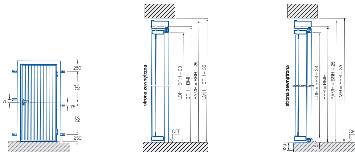
Rozmieszczenie kotew
