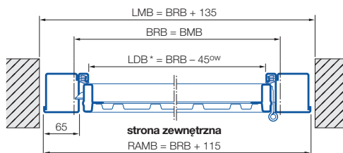
Montaż w otworze / otwieranie na zewnątrz
