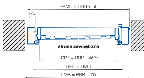
Montaż w otworze / otwieranie do wewnątrz
