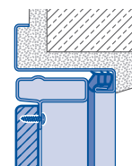
Widok: układ wypełnienia w ramie
