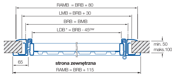
Montaż od zewnątrz / otwieranie na zewnątrz
