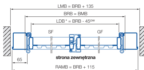
Montaż w otworze / otwieranie na zewnątrz
