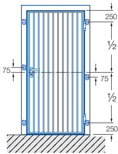
Rozmieszczenie kotew
