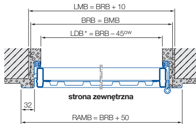
Montaż od zewnątrz / otwieranie na zewnątrz
