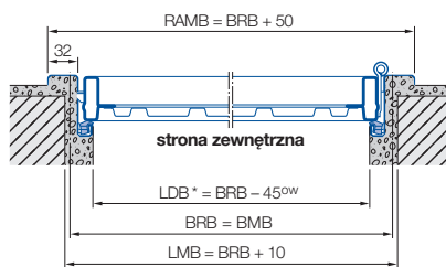
Montaż od wewnątrz / otwieranie do wewnątrz
