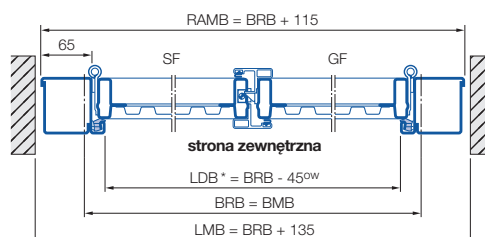
Montaż w otworze / otwieranie do wewnątrz
