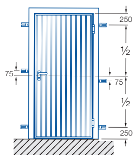
Rozmieszczenie kotew
