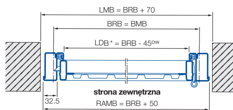
Montaż w otworze / otwieranie na zewnątrz
