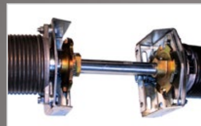
MZS – zabezpieczenie przed opadnięciem bramy w wypadku pęknięcia sprężyny
